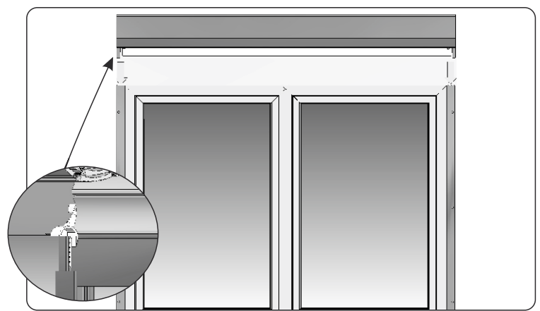
14. Präzise den Kasten auf die Führung verschieben, dabei die Bolzen der Seiten in den Oberteil der Führungen sorgfältig einführen, den korrekten Einbau der Einlaufrichter von Federn prüfen.
