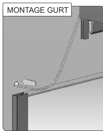
13. Den Gurt (Schnur oder Leitung) durch die Öffnung in den Innenbereich des Gebäudes verlegen.
