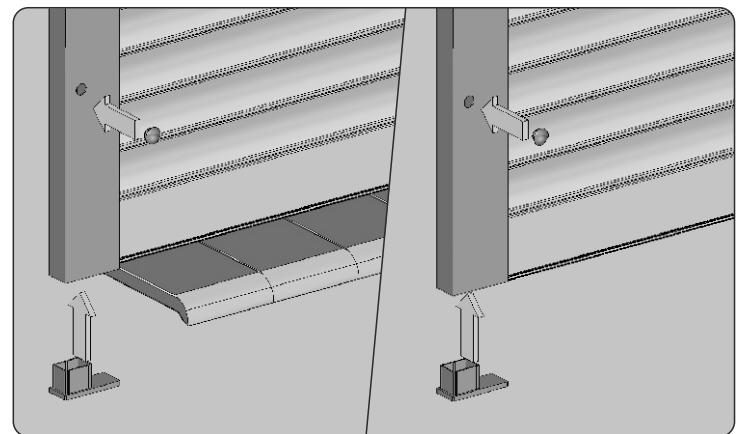
16. Sich vergewissern, dass der Rollläden sachgerecht (waagrecht und senkrecht) befestigt ist. Stifte in Führungen verschrauben und dann Abdeckungen einlegen und bei Bedarf untere Abdeckungen der Führungen einbauen. Die sachgerechte Funktion des Rollladens prüfen. Die sachgerechte Funktion der automatischen Riegel oder des Verschlusses prüfen, bei Bedarf regeln.
