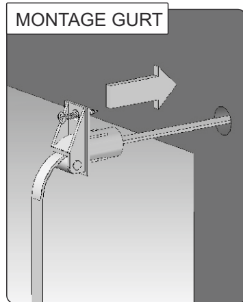
15. Den Gurt oder den Schnur durch die Durchführung führen und dann die Durchführung mit dem Spreizdübel an der Wand befestigen.
