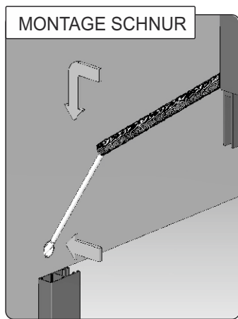
13. Den Gurt (Schnur oder Leitung) durch die Öffnung in den Innenbereich des Gebäudes verlegen.
