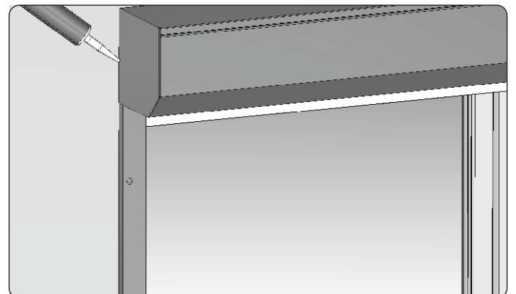
18. Es empfiehlt sich nach dem Einbau die oberen und unteren Spalten zwischen der Mauer und dem Rollladen mit Silikon füllen, um zusätzliche Abdichtung und Wasserschutz sicherzustellen.
