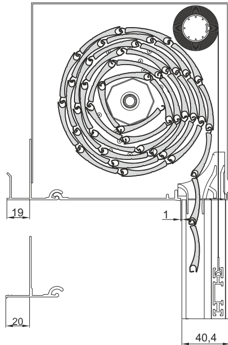
Volet roulant IT2000® avec moustiquaire
