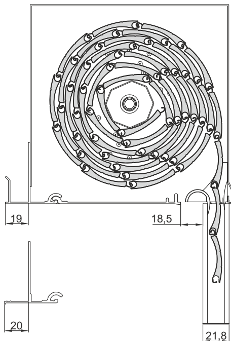
Volet roulant IT2000®
