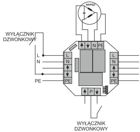
Rys. 2 Schemat podłączenia sterownika SIR z wyłącznikiem dzwonkowym
