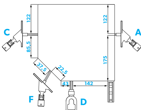
SKRZYNKA 300 FI 60
