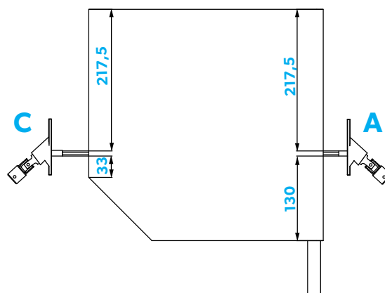
SKRZYNKA 350 FI 70
