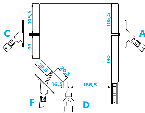
SKRZYNKA 300 FI 70
