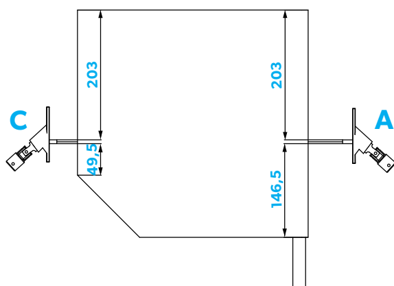
SKRZYNKA 350 FI 60
