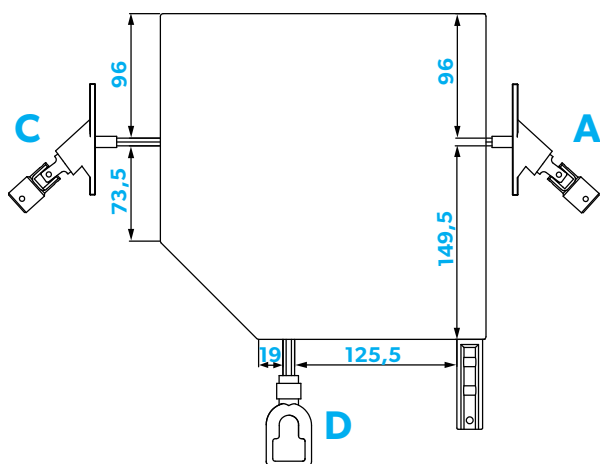
SKRZYNKA 250 FI 60
