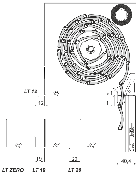
Volet roulant IT2000® avec moustiquaire
