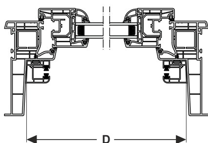
DISTANCE ENTRE LES COULISSES NRR-020
